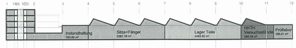
Abb.6: Längsschnitt
