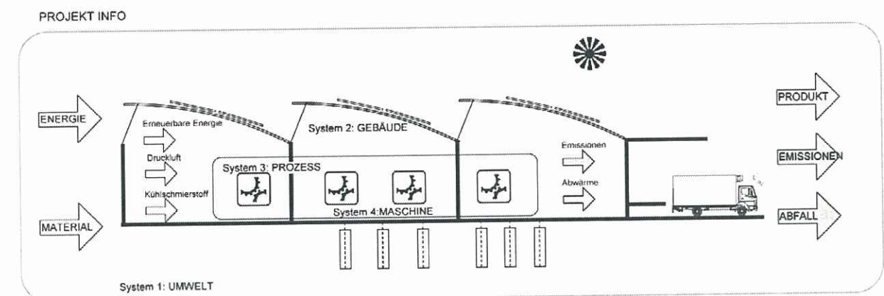
Abb. 4: Projekt INFO – Modell für Integrale Simulation
