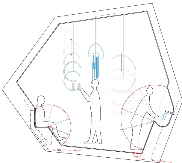
Systemschnitt, Nasszellenmodul / System section, sanitary block module
