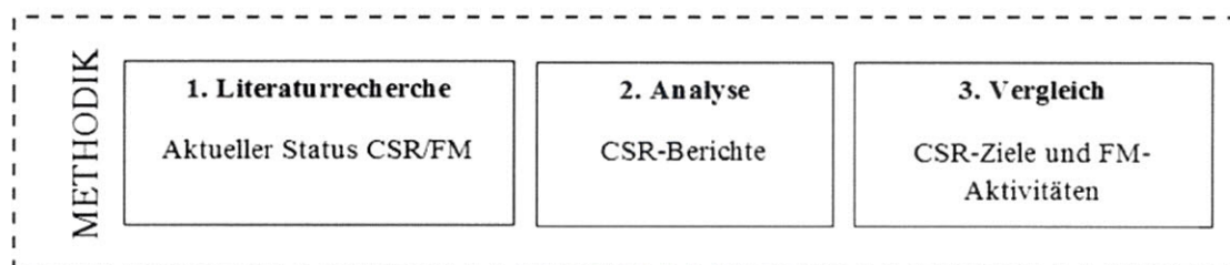
Abb. 1: Methodische Vorgehensweise
