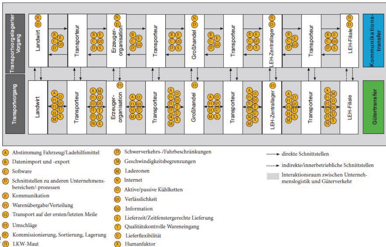
Abbildung 23: Systematik zur Schnittstellenfindung und -zuordnung für die Branche Frischgemüse
