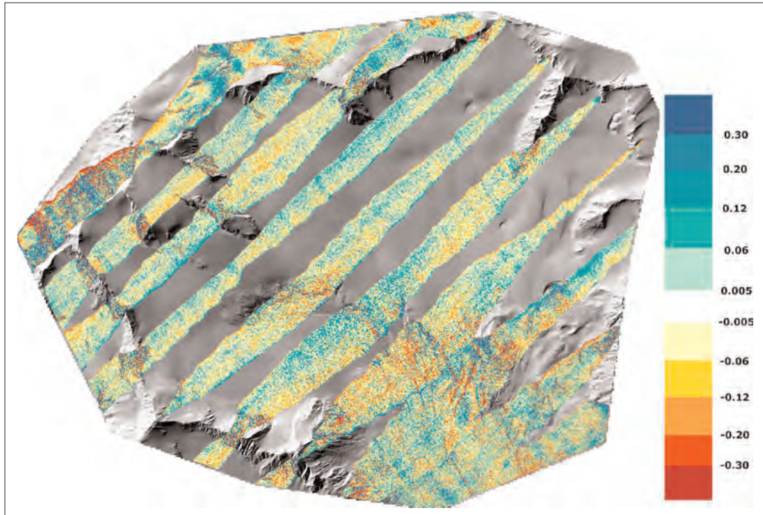
Bild 6 – Streifendifferenzen nach Georeferenzierung (Skala in m).
