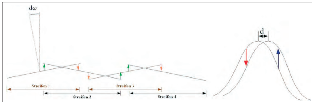
Bild 5 – Resultierende Streifendifferenzen aufgrund von konstantem Querneigungsfehler d\omega und Lageverschiebung d .
