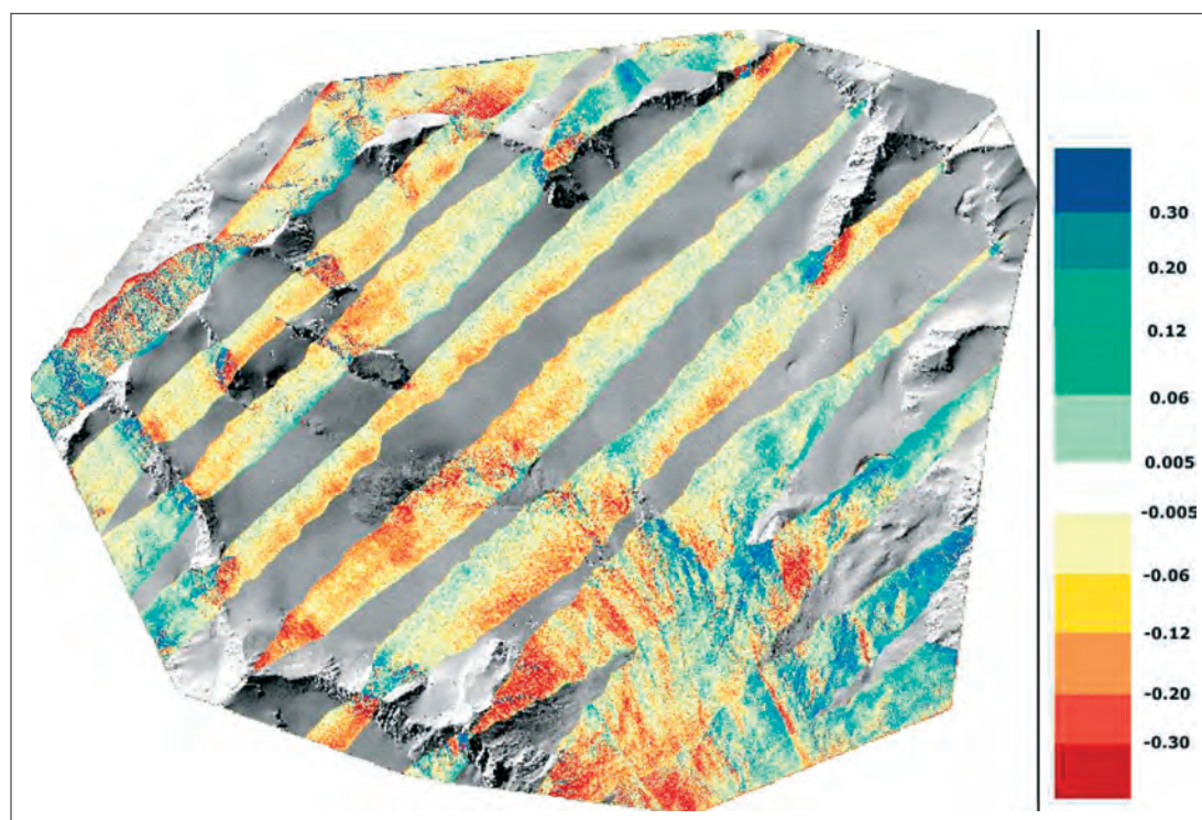
Bild 4 – Streifendifferenzen vor Georeferenzierung (Skala in m).
