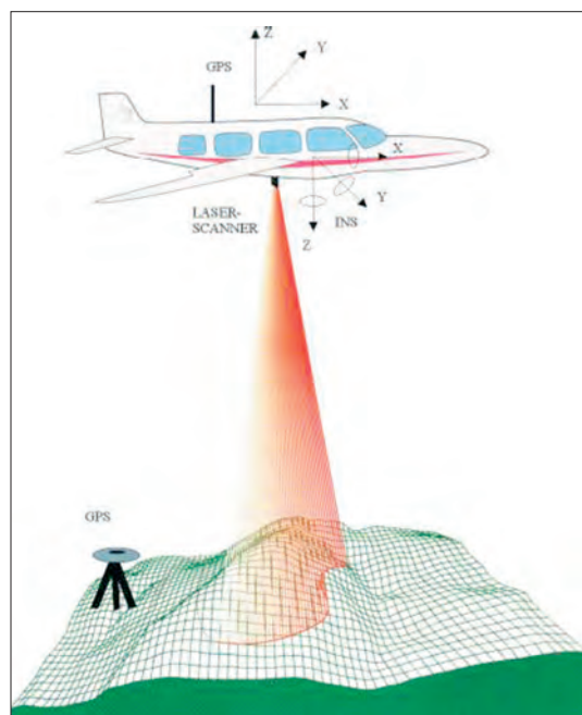
Bild 1 – Prinzip des flugzeuggetragenen Laserscannings. (Graphik in Anlehnung an TopScan 2005)
