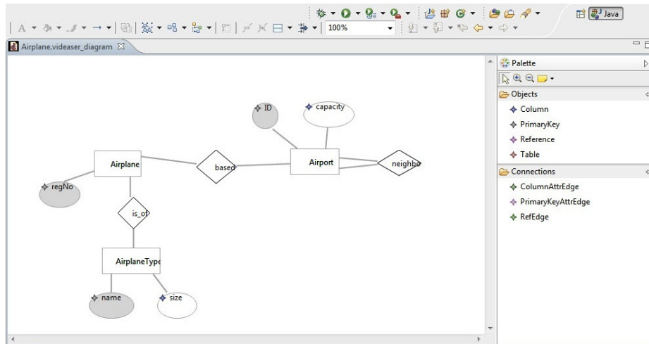
Fig. 3. Screenshot of the ER editor.
