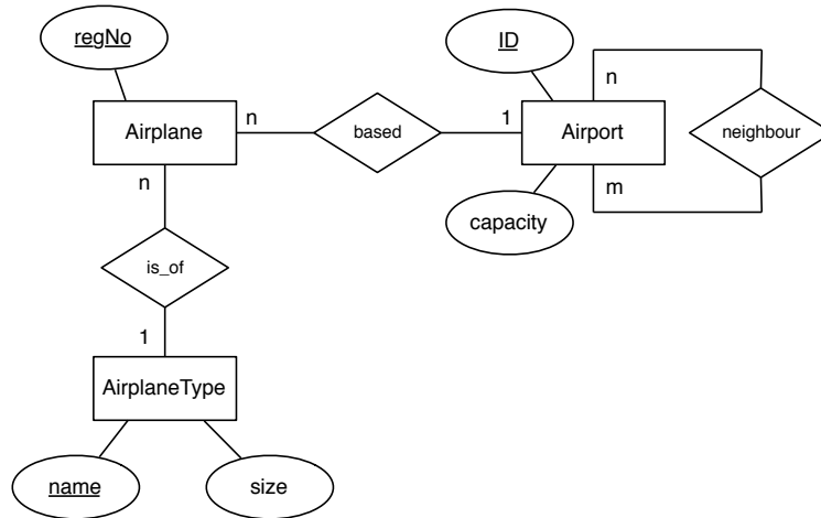
Fig. 2. Example of an ER diagram.
