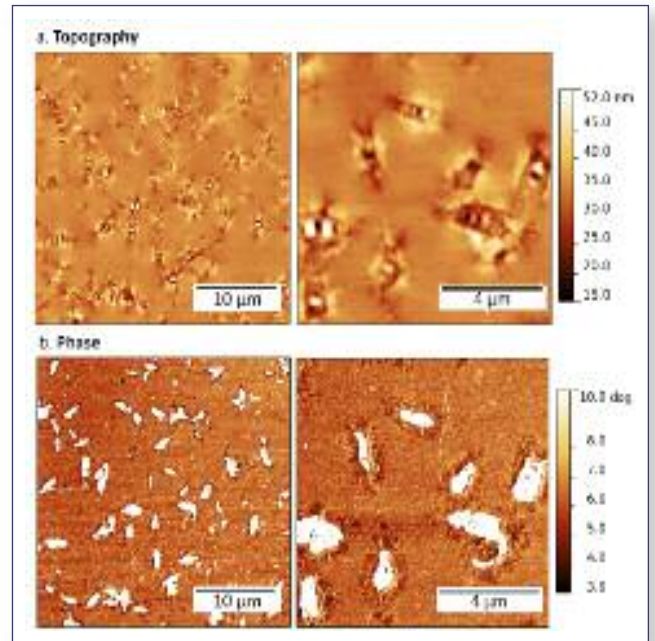
FIG. 6 Microstruttura del campione ricostruito con aggiunta ai maltini dell'8,73% di asfalteni.
