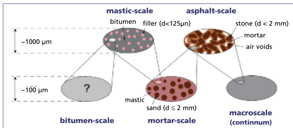
FIG. 1 Modello multi-scala del conglomerato bituminoso
