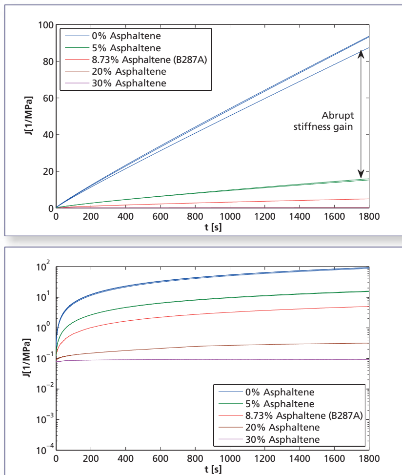
FIG. 3 A-B Comportamento al creep (prove CR) di campioni di bitume a 5°C.
