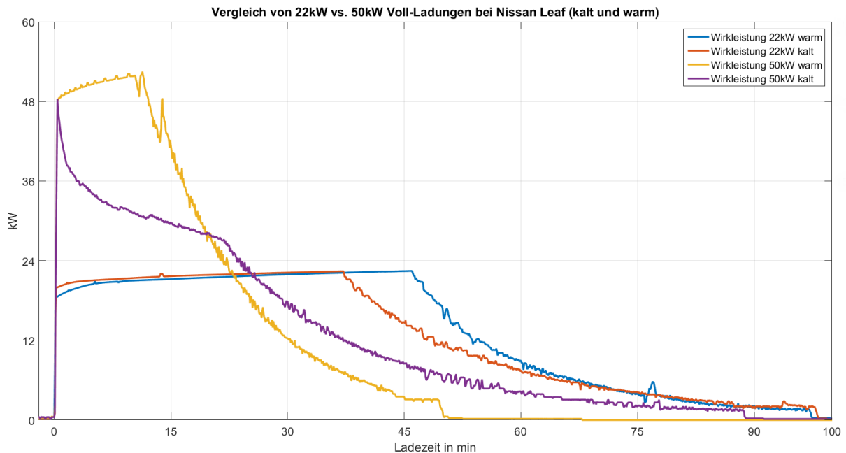
Abbildung 9: Vergleich von verschiedenen Vollladungen eines Nissan Leaf mit unterschiedlichen Ladeleistungen und Batterietemperaturen
