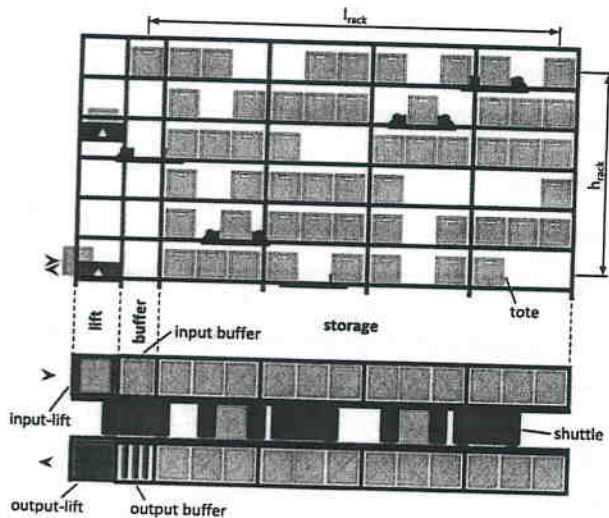
Abbildung 1. Aufbau des untersuchten Shuttle-Systems [Kar14]
