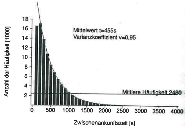
Abbildung 6. Häufigkeitsverteilung der Zwischenankunftszeiten des Lifes bezogen auf eine einzelne Regalebene für ein Regal mit 56 Ebenen
