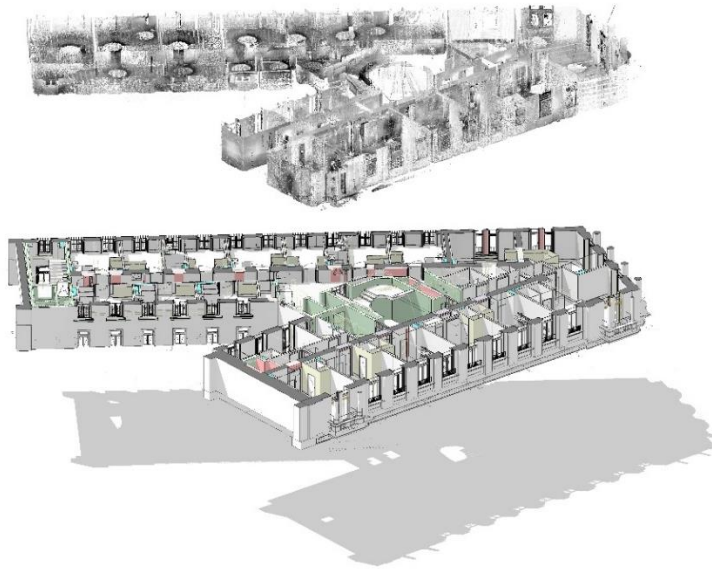
Bild 3: Bestandsaufnahme mittels 3D-Laserscan und abgeleitetes BIM-Modell 16
