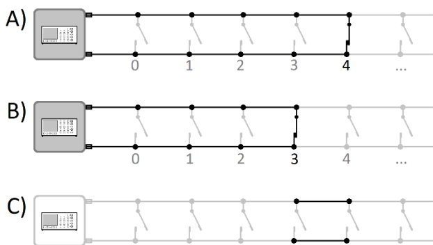
Abbildung 13. Analysegerät mit elektrischen Leitern, die Messknoten Index 0 bis 4 sind vereinfacht als Schalter dargestellt
