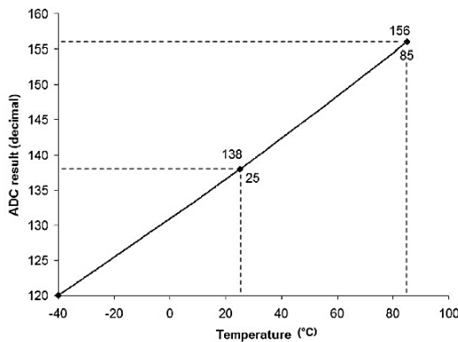
Abbildung 12. Temperaturkalibrierung PIC10LF322 [Mic13]
