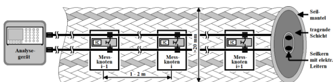
Abbildung 7. Prinzipische Skizze des Messsystems
