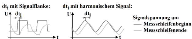
Abbildung 14. Bestimmung der Signalverschiebung dt_i
