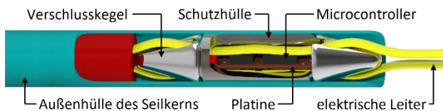
Abbildung 9. Messknoten mit Schutzhülle und elektrischen Leitern in Schnittansicht
