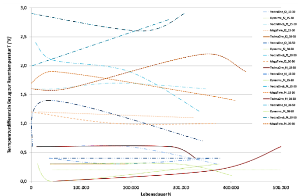
Abbildung 4. Erwärmung durch innere Reibung im Betrieb bei verschiedenen Seilen (Material und Machart) [Weh17]
