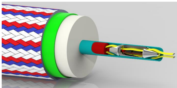
Abbildung 8. Schnittansicht der im Seilkern eingebetteten elektrischen Leiter mit einem Messknoten
