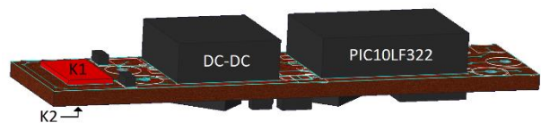
Abbildung 11. Layout und 3D-Modell der Messknoten-Platine
