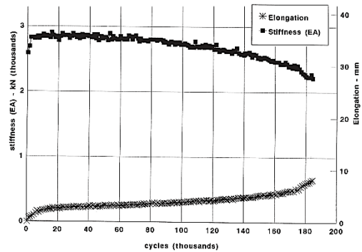
Abbildung 3. Änderung der Steifigkeit und Dehnung eines LCP-Seils über dessen Lebensdauer [BC98]
